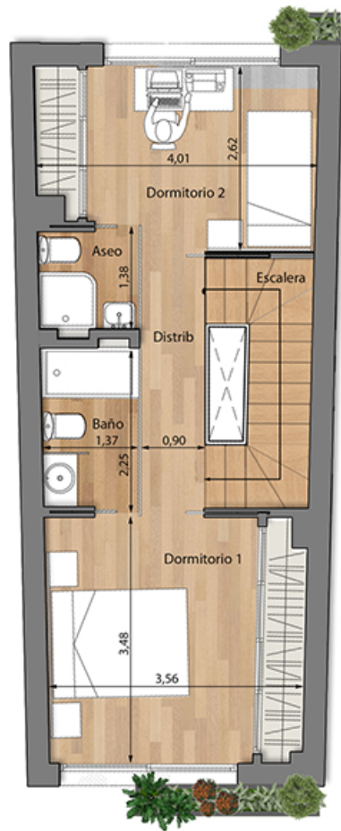
Planta Alta
