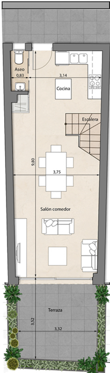
Planta Baja
