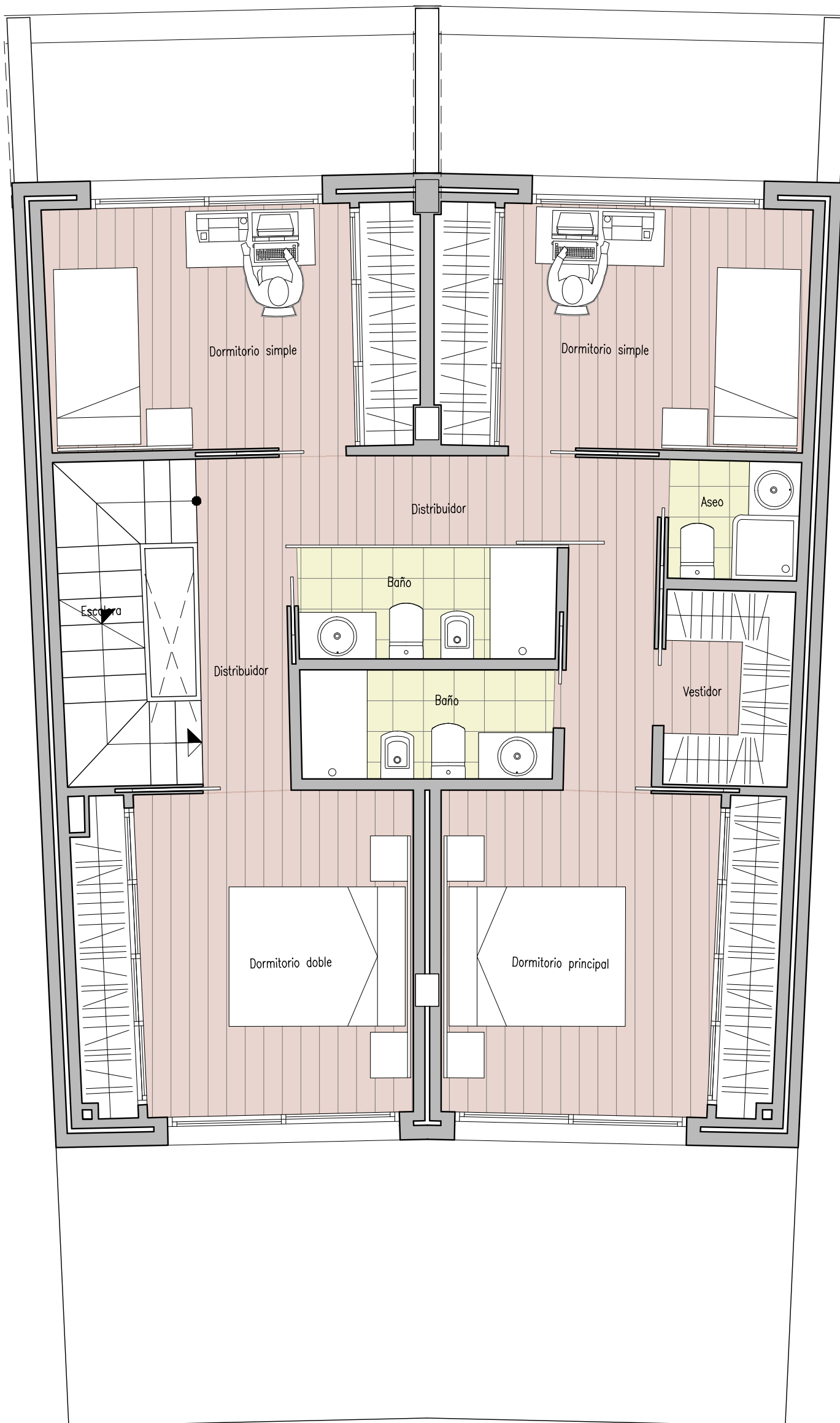
PLANTA PRIMERA
